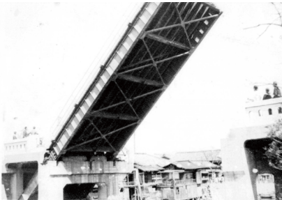
開閉橋
